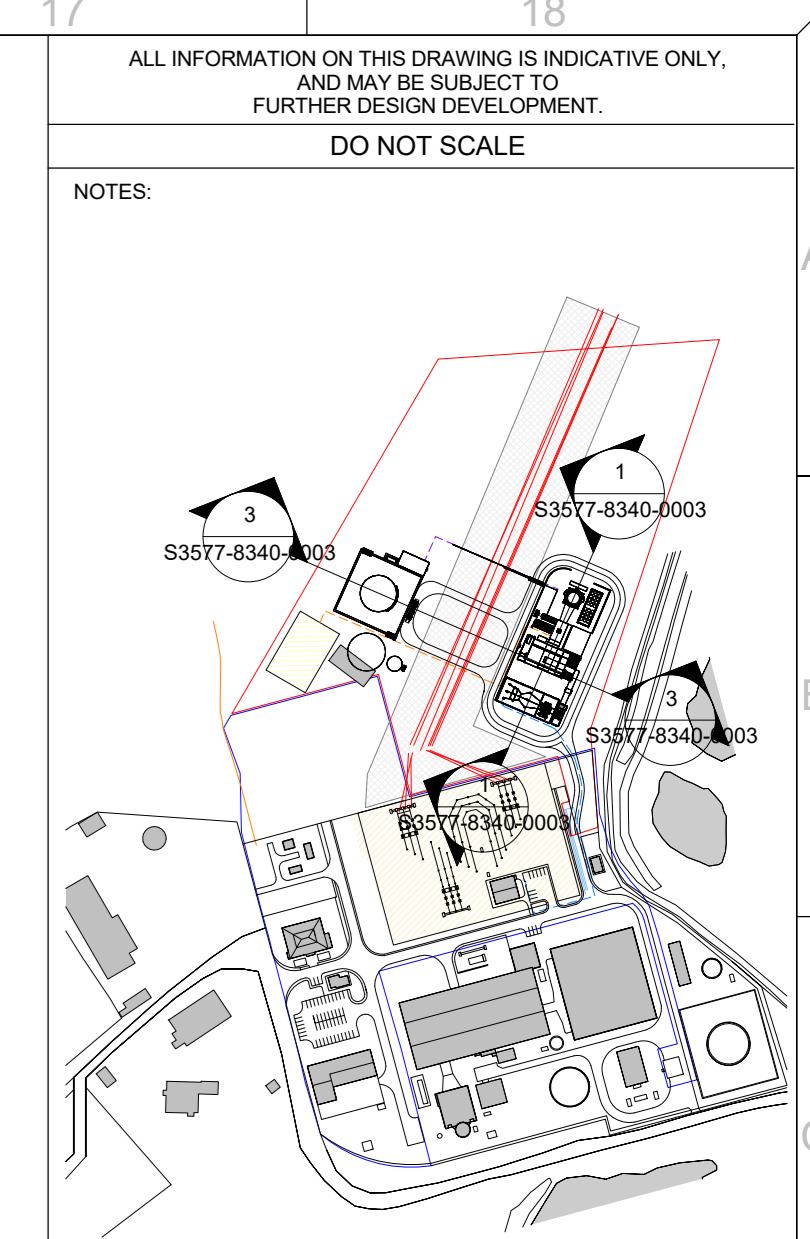
OCGT Key Plan 1 : 5000
